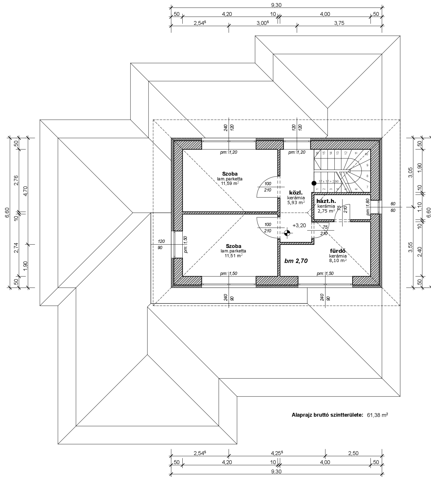
Emeleti alaprajz
